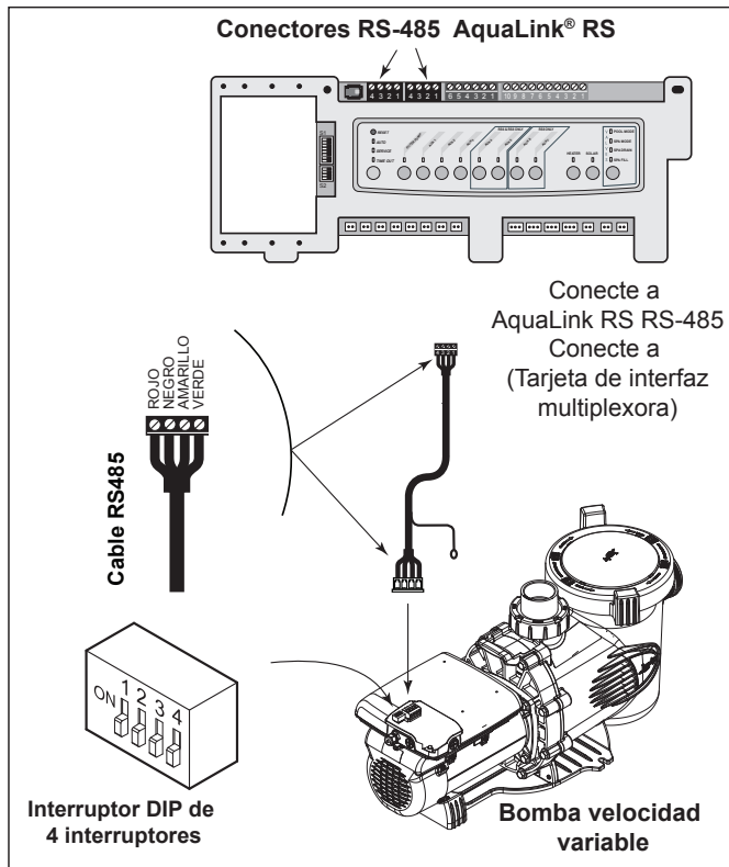
Figura 5A. Cableado del controlador AquaLink RS o AquaLink PDA a la ePump, Motor Regal Beloit
