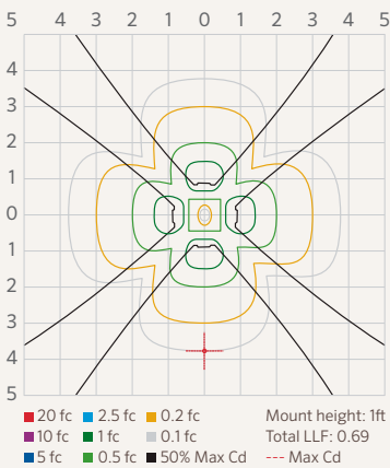
FC ZDC ISOFOOTCANDLE PLOT
