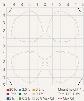
FC 9LED ISOFOOTCANDLE PLOT
