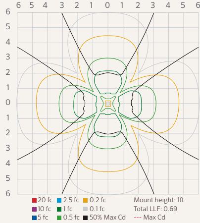
FC 9LED ISOFOOTCANDLE PLOT
