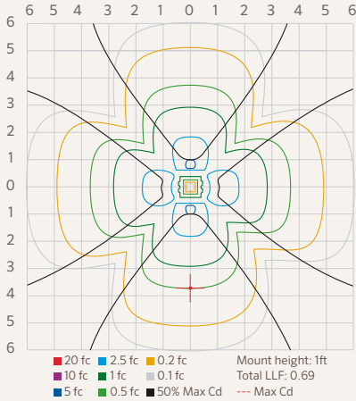
FC ZDC ISOFOOTCANDLE PLOT
