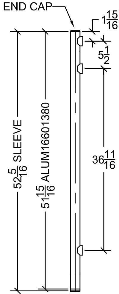
QTY: 2 BOTTOM END CAP FP-2448-CEP
