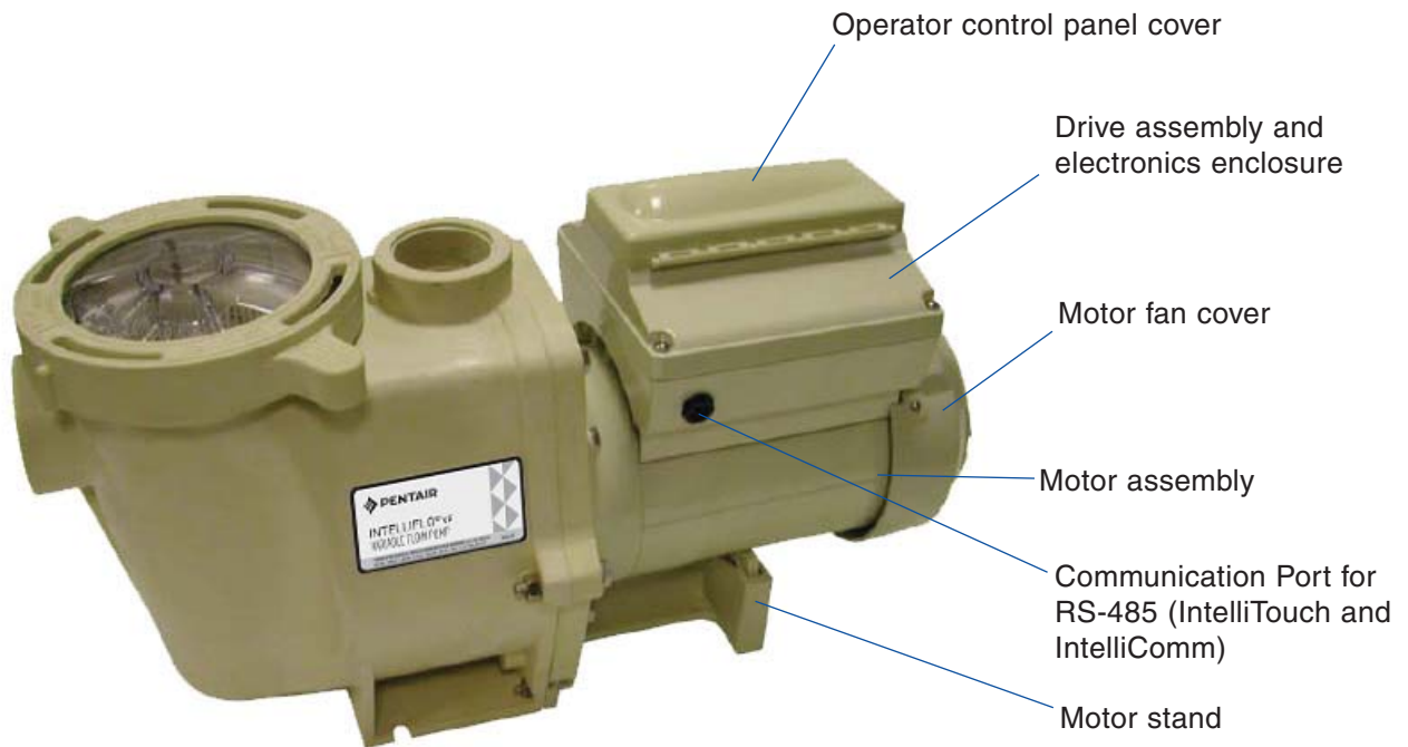
IntelliFlo VF Motor Assembly
