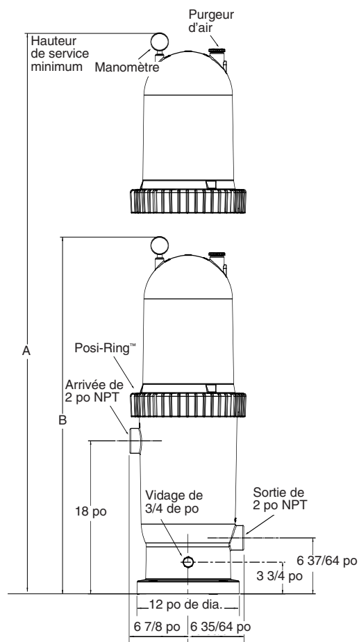
FIGURE 1 – Dimensions en pouces (en mm)
